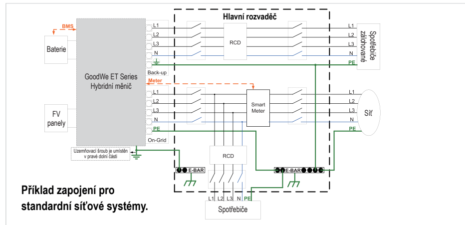
Příklad zapojení pro Austrálii a Nový Zéland.
